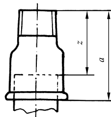
异径内外丝接头 M4(246)
